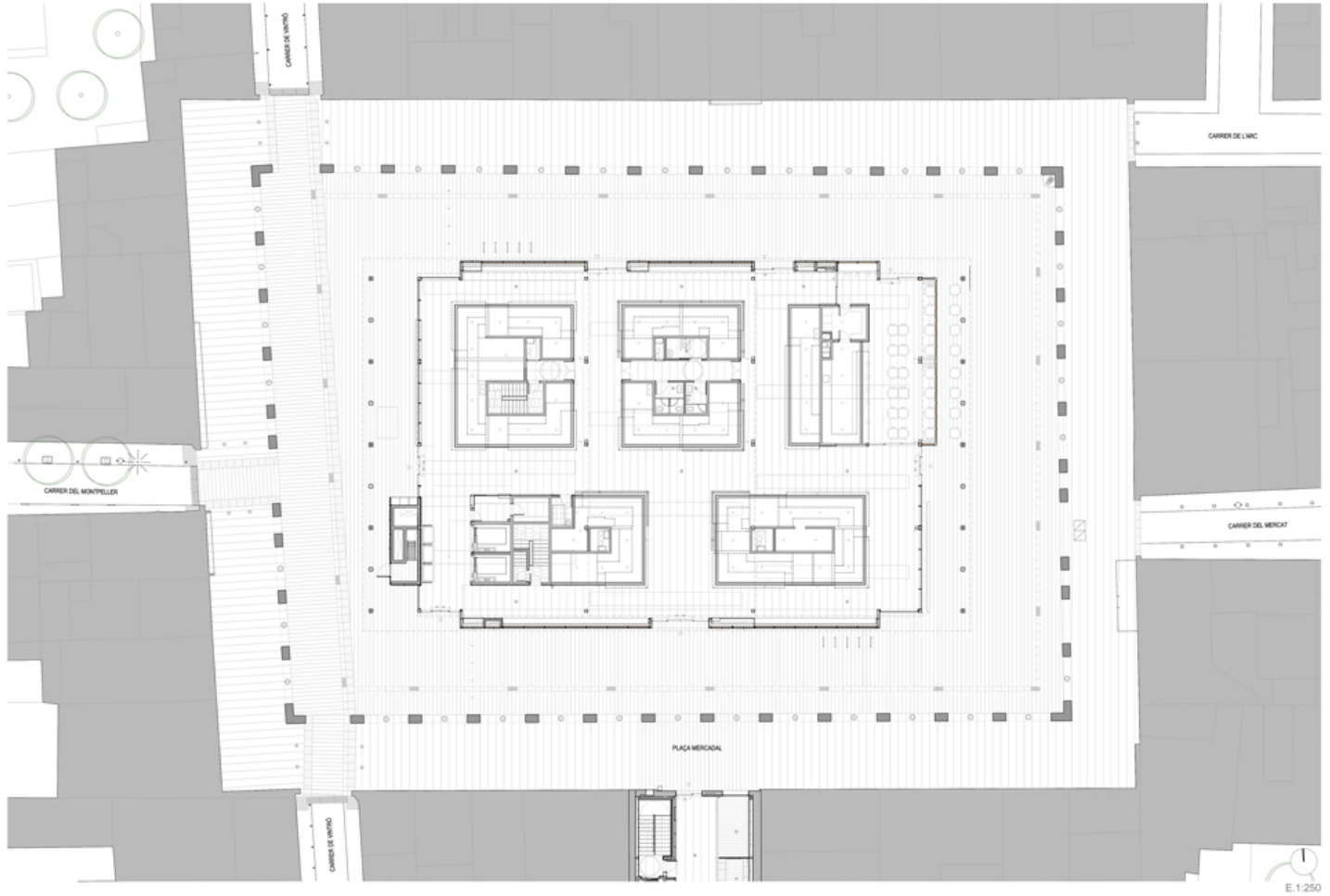
PLANTA BAIXA I PROJECTE DE REMODELACIÓ DEL MERCAT DE SANT ANDREU A BARCELONA
