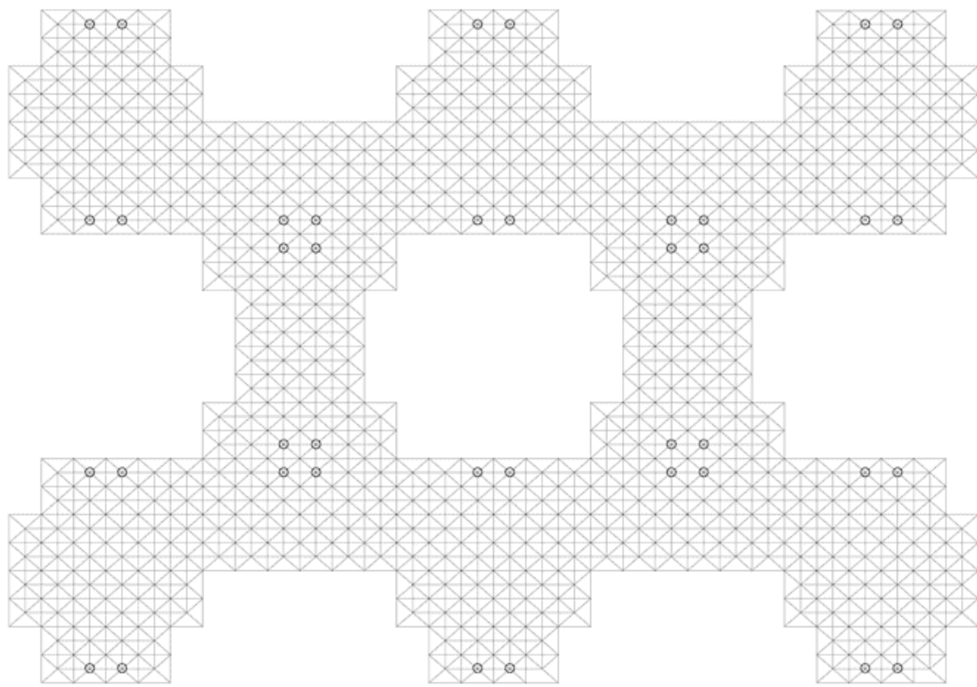
SPACEFRAME
