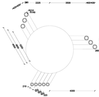
平面圖 1:50 plan 1m 1:50
